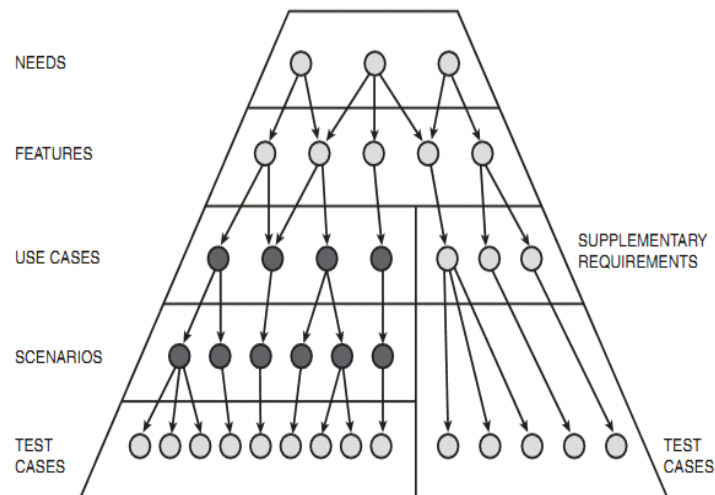
Hình 6.1 Kim tự tháp yêu cầu
